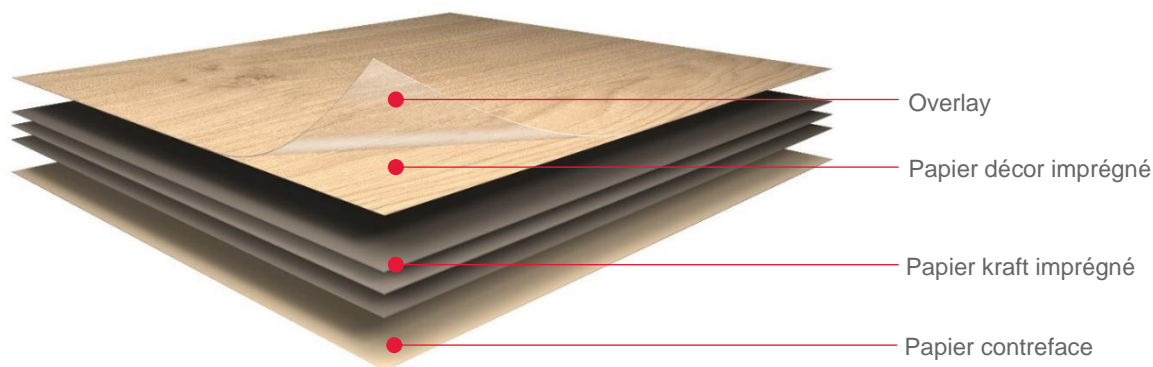
Structure de stratifié MED (épaisseur nominale de 0,8 mm)
