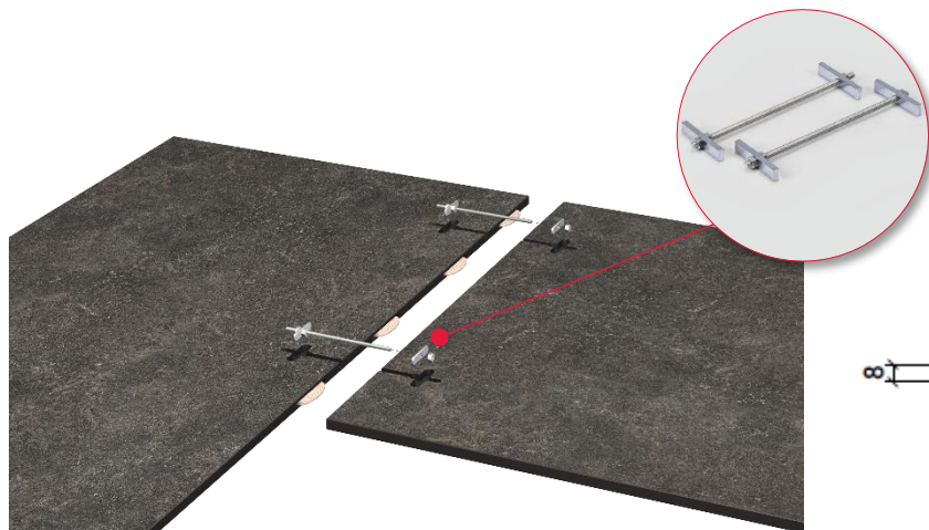
Фигура 1: Съединяване на кухненски плотове от компакт 12 мм съединителя – дълбочина 8 мм
