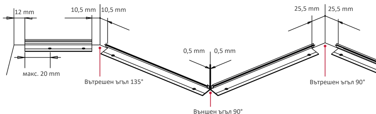
Основен профил
