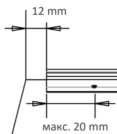
Крепезни размери основен профил
