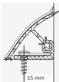
Закрепване основен профил
